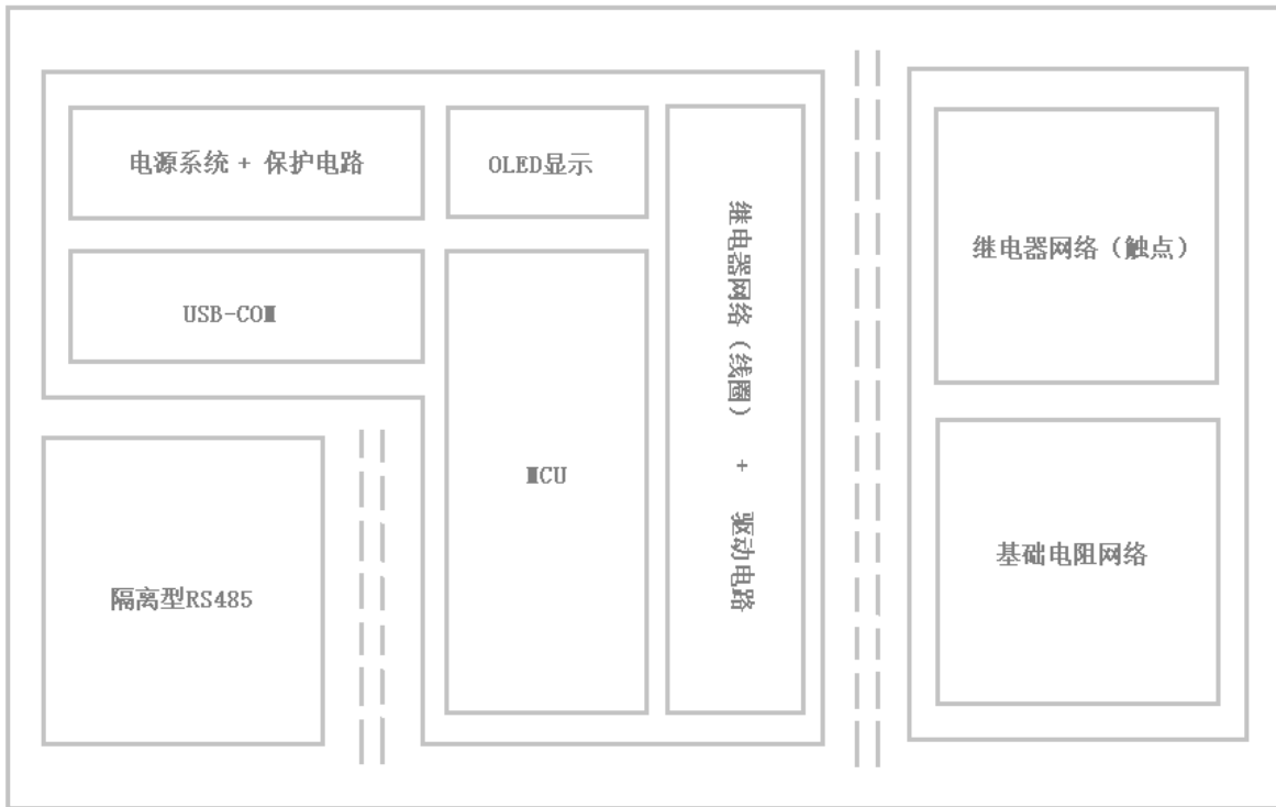
上图：RM550 模块系统框图
