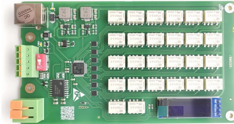
上图：模块 TOP 视图（HW v1.1）
