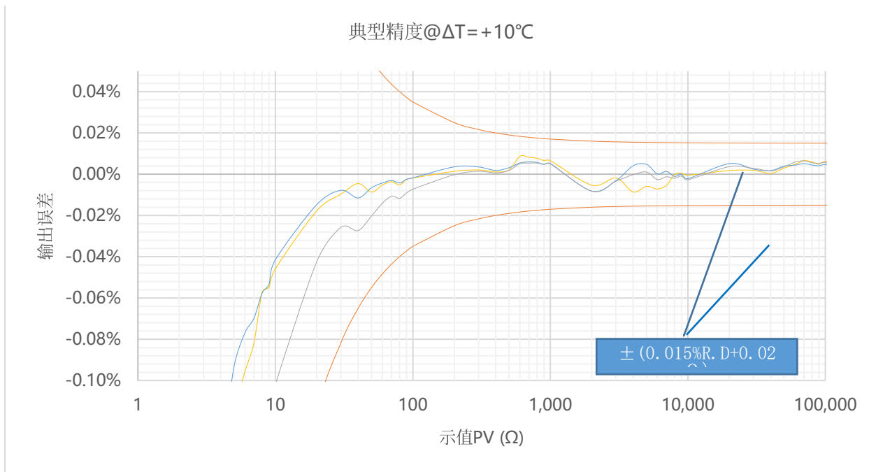
上图：精度是基于数个样品在 T_{cat}+10^\circ\text{C} ( 34^\circ\text{C} ) 条件下测试的结果汇总
