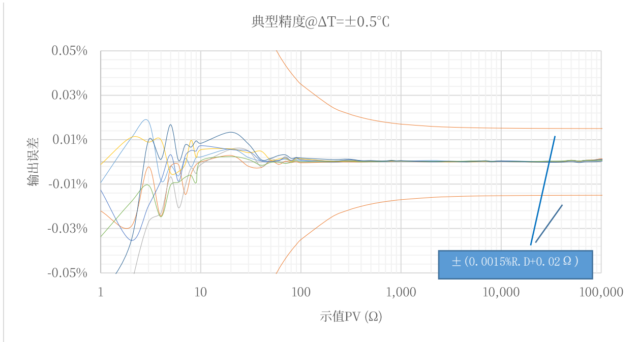
上图：精度是基于数个样品在恒温箱内（温度变化区间： T_{cat}-0.5^\circ\text{C} \sim T_{cat}+0.5^\circ\text{C} ）测试的结果汇总
