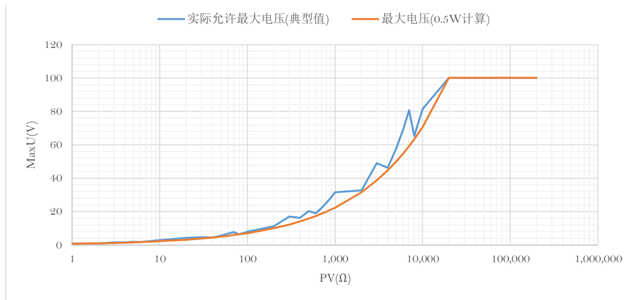
上图：BMR-L 基础电阻的额定功率是 0.5W，而实际上对于绝大多数的输出值（PV），其额定功率通常在 0.5W 至 1W 之间。用户可根据串口实际返回的 MaxU 来使用；简化起见，也可一律按照 0.5W 根据公式 \text{MaxU} = \sqrt{\text{PV} \times 1} 计算出的额定电压来处理。需要注意的是，输出电阻两端最大施加电压不能超过 100V。
