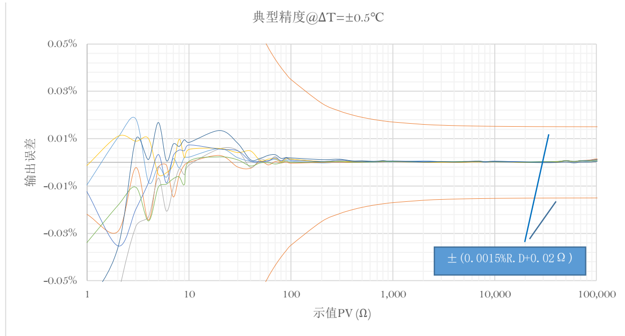
上图：精度是基于数个样品在恒温箱内（温度变化区间： T_{cal}-0.5^\circ\text{C} \sim T_{cal}+0.5^\circ\text{C} ）测试的结果汇总
