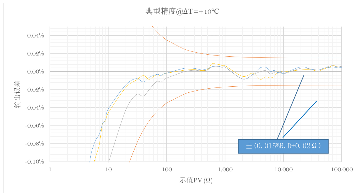
上图：精度是基于数个样品在 T_{cal}+10^\circ\text{C} ( 34^\circ\text{C} ) 条件下测试的结果汇总
