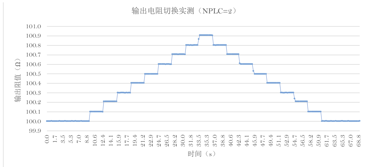
上图：输出由 100Ω 以步进 0.1Ω 递增至 100.9Ω，再递减至 100Ω，每一测点停留 3s，万用表设置 NPLC=2
